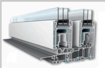
VekaSlide 82 hefschuifraam Uf-waarde: 1,4 W/m 2 .K.
