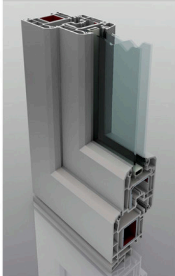
TopLine AD 5- kamerprofiel: Uf-waarde: 1,3 W/m 2 .K.
