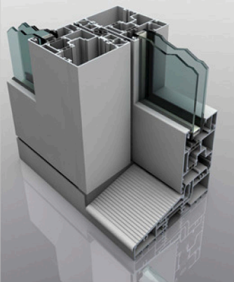
Standaard: Uf-waarde: 3,0 W/m 2 .K
